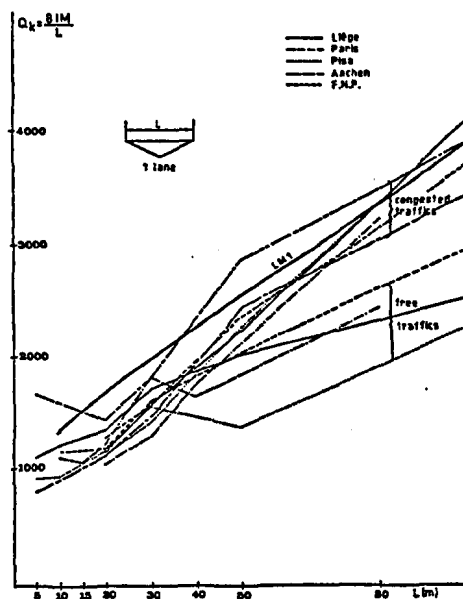
Fig. 7. Target values - M_o - 1 lane
