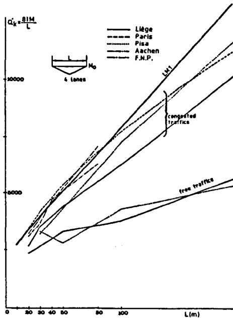
Fig. 10. Target values M_0 - 4 lanes
