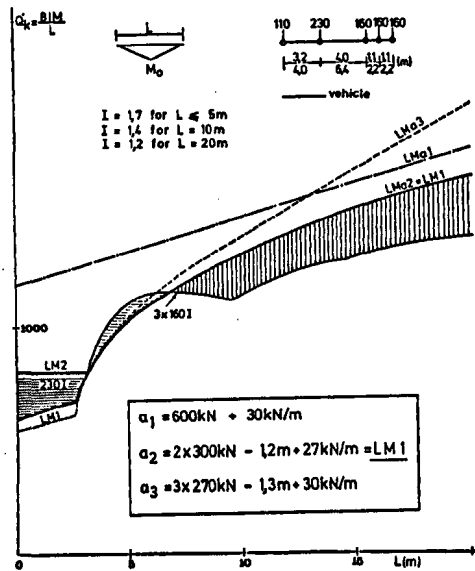
Fig. 8a. Target values - M_0 - Local effects
