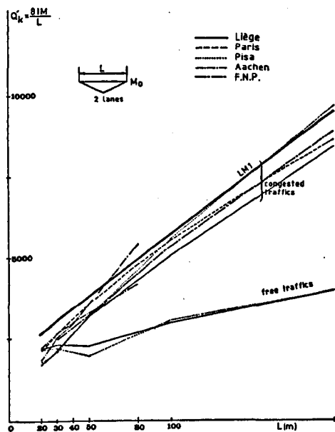
Fig. 9. Target values M_0 - 2 lanes
